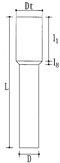
図-別-7 拡頭ぐい
