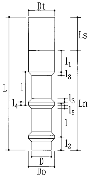
図-別-5 複合節ぐい
