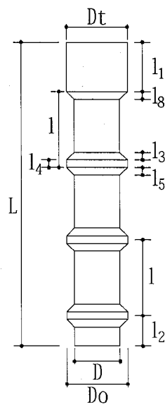
図-別-3 拡頭節ぐい (節部径タイプ)
