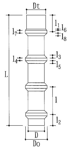
図-別-4 拡頭節ぐい (中間径タイプ)
