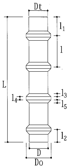
図-別-2 節ぐい
