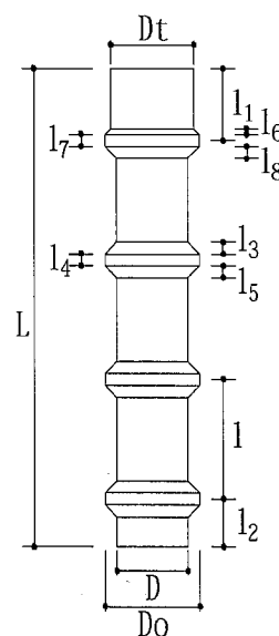
図-別-4 拡頭節ぐい (中間径タイプ)
