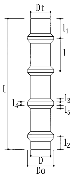
図-別-2 節ぐい
