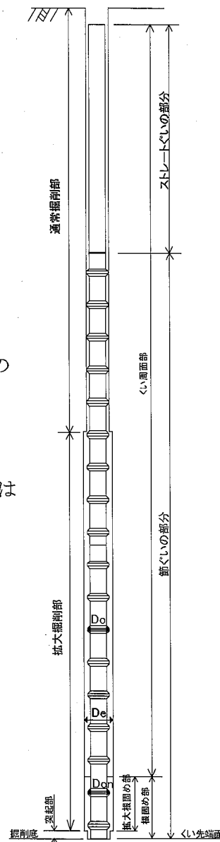
図・別-1 基礎ぐい設置概要図
