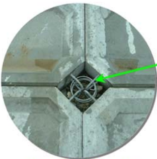
連結部（モルタル充填前）
