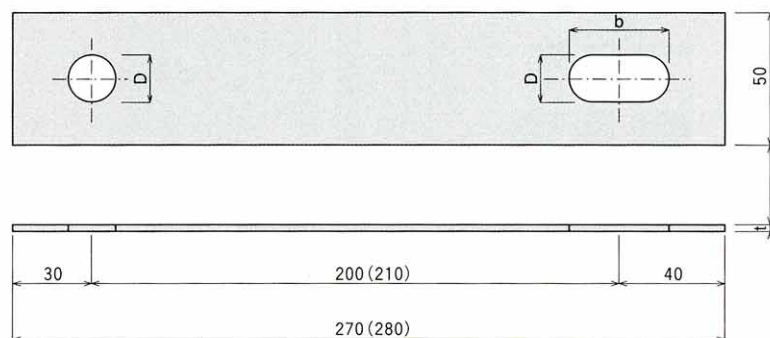
緊結プレート 単位：mm
