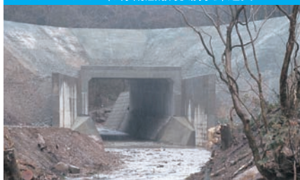
北陸農政局佐渡農業水利事業所 新潟県佐渡市 6200B×4900H(3分割底版現場打ち)延長24.1m
